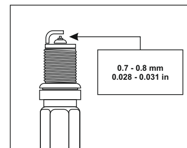
Рисунок 31 – Установка свечи
