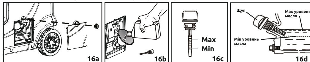
Рисунок 16 - Уровень масла
