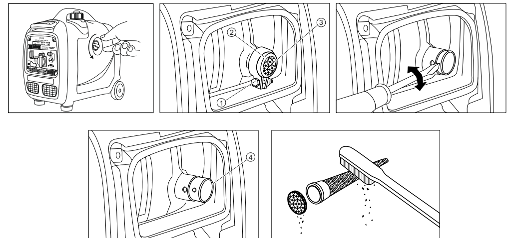
Рисунок 11 – Искрогаситель
