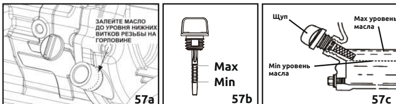
Рисунок 57 - Уровень масла
