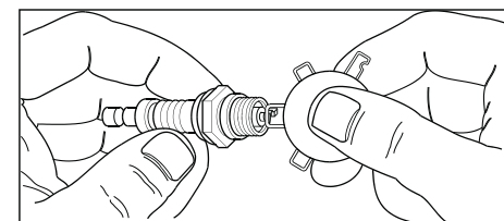
Рисунок 9 – Установка свечи
