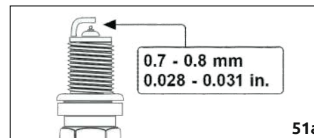
Рисунок 51 – Установка свечи
