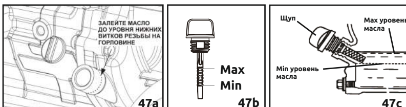
Рисунок 47 - Уровень масла
