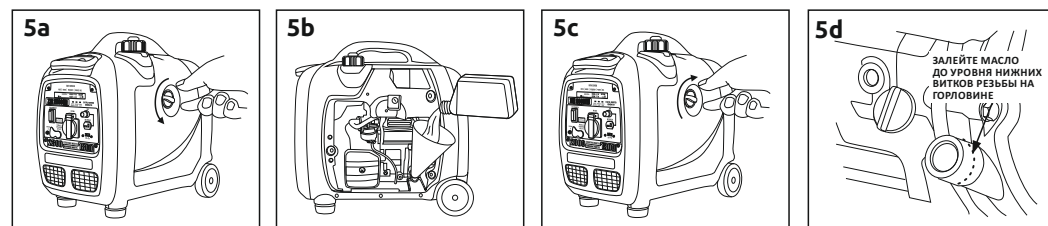
Рисунок 5 - Уровень масла
