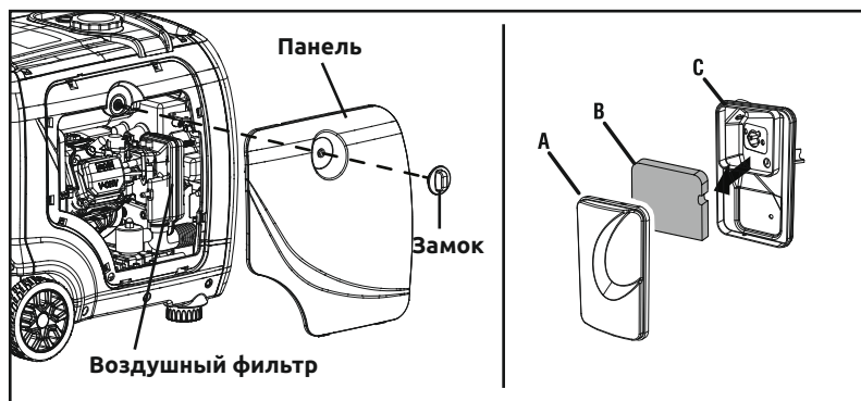
Рисунок 21 – Воздушный фильтр
