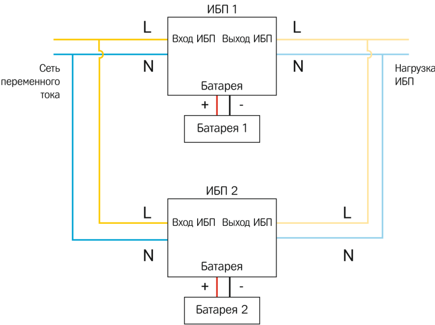
Схема параллельного соединения ИБП
