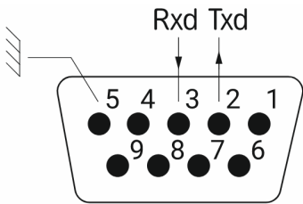
Порт RS-232 на ИБП
