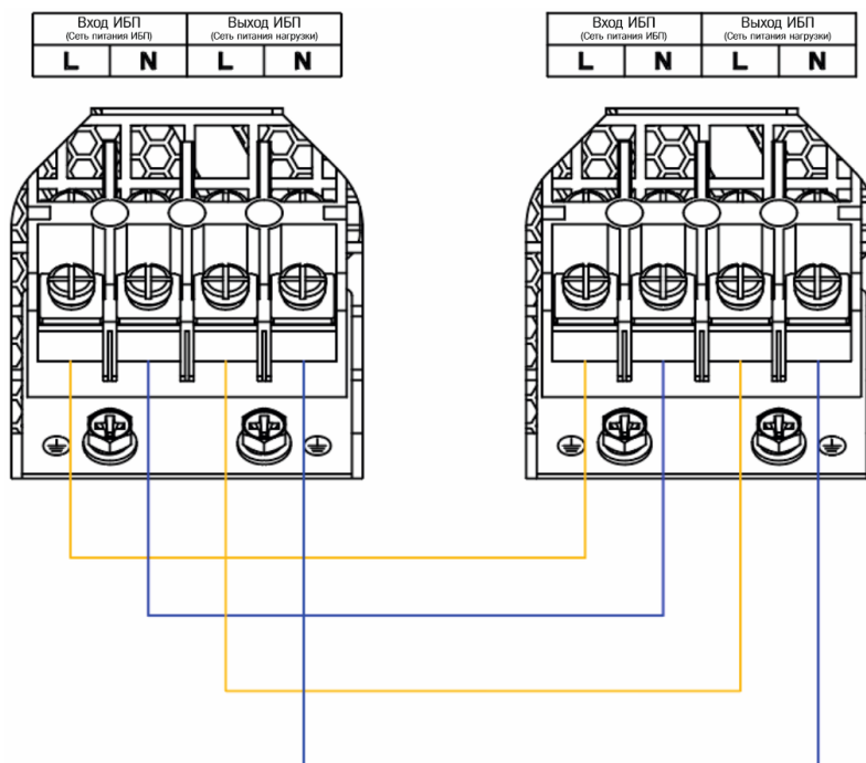
Подключение коммуникационных кабелей RS-232
