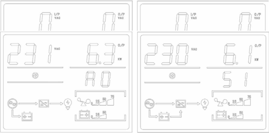
Параллельный режим, в нормальном состоянии нагрузки
